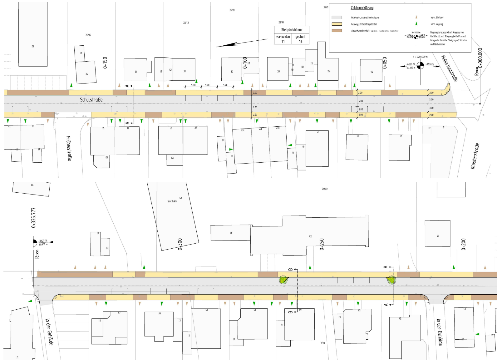
Lageplan
